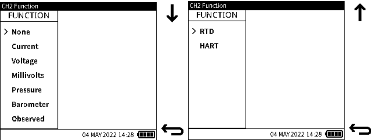
图 6-4：通道 2 功能
