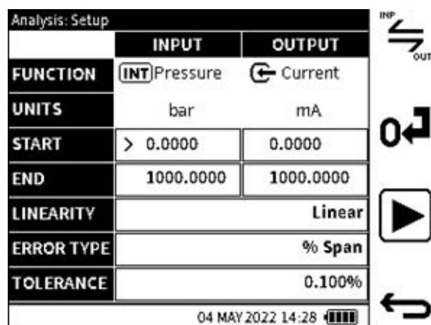
图 11-2：分析功能屏幕
