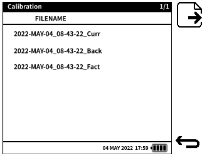
图 15-1：校准文件屏幕
