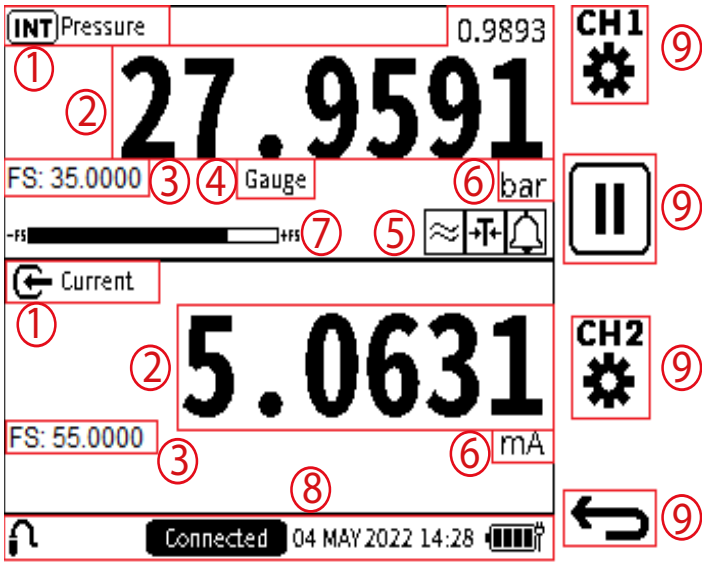
图 6-1：校准器任务屏幕
