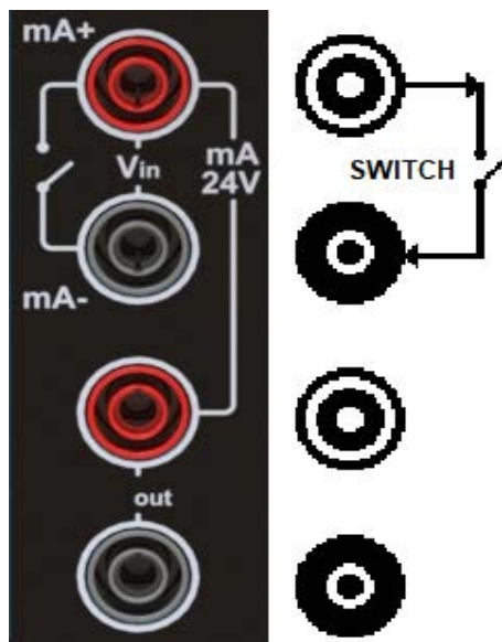
图 8-1：高度开关测试连接
