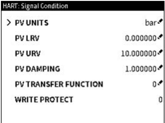
图 13-4: 信号条件屏幕
