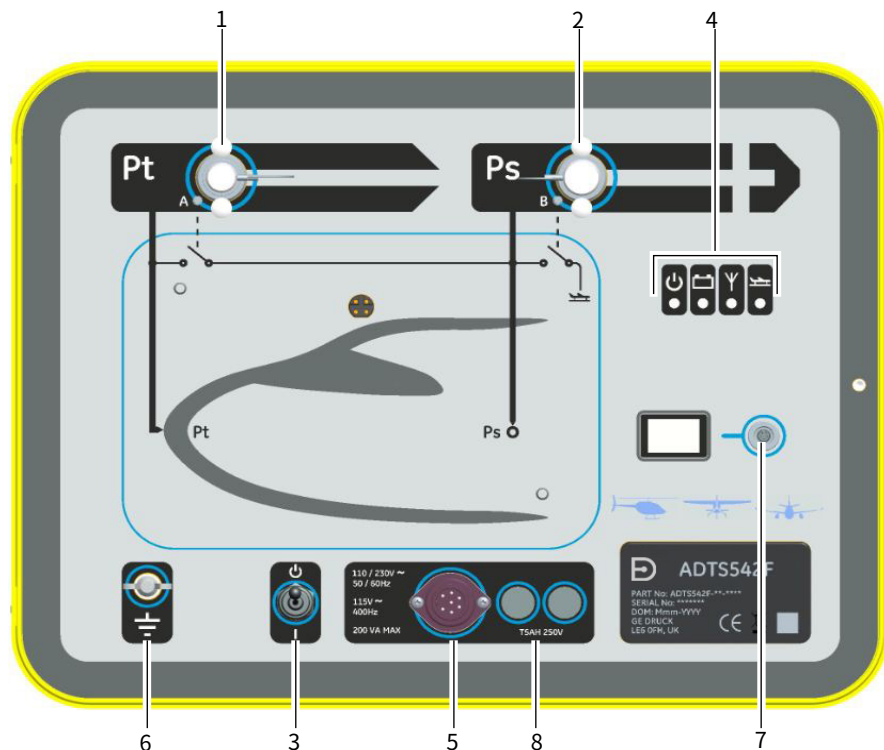
图 6: ADTS542F 前面板
